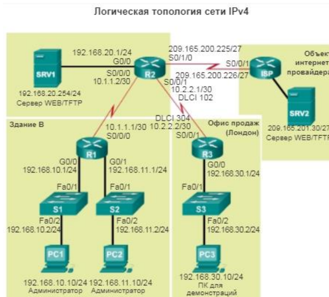
Рисунок 1. Пример логической топологии сети
